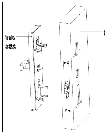
4.前锁安装示意图
