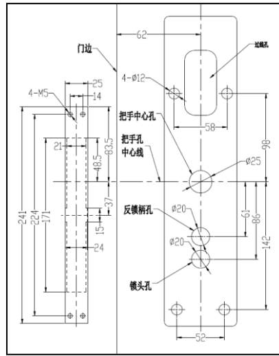
2.锁芯, 锁体安装孔示意图
