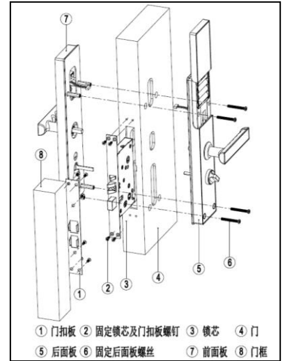
3.锁芯, 锁体安装总图
