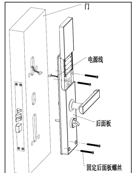
5.门扣板安装示意图
