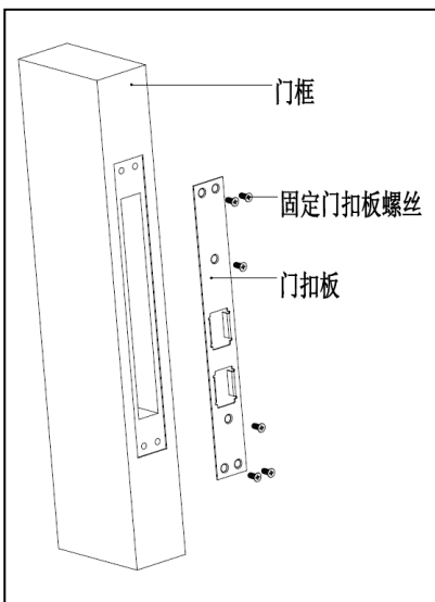
3.后门扣板安装示意图
